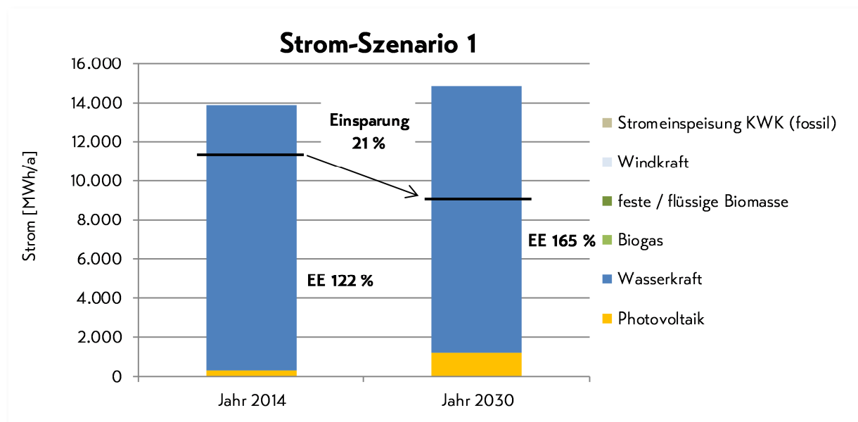
Abbildung 23: Strom-Szenario 1
