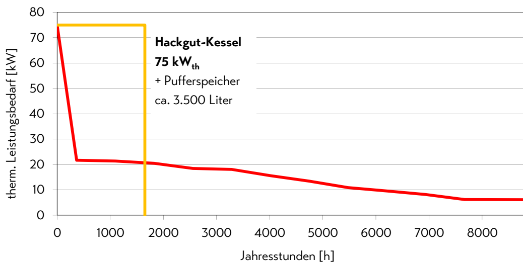
Abbildung 28: Energieversorgungsvariante 1.2
