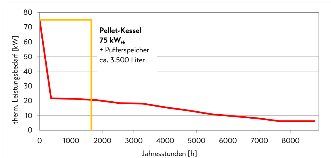
Abbildung 27: Energieversorgungsvariante 1.1
